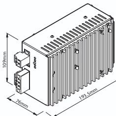
Optional DIN rail mount approx. 1.0 kg
